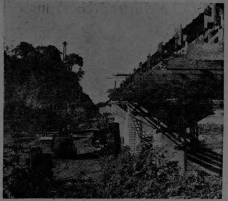
El magnífico puente sobre el Río Terraba en Palmar Sur, va poco a poco tomando forma, conforme el esfuerzo humano se prolonga. La presente gráfica muestra el estado actual de la construcción la que ya nos da una idea de la magnitud de la obra que unirá dentro de un año, más o menos, las poblaciones de Palmar Norte y Palmar Sur. Este puente, construido sobre la Carretera Interamericana, será el de mayor extensión en el tramo centroamericano de la misma.
